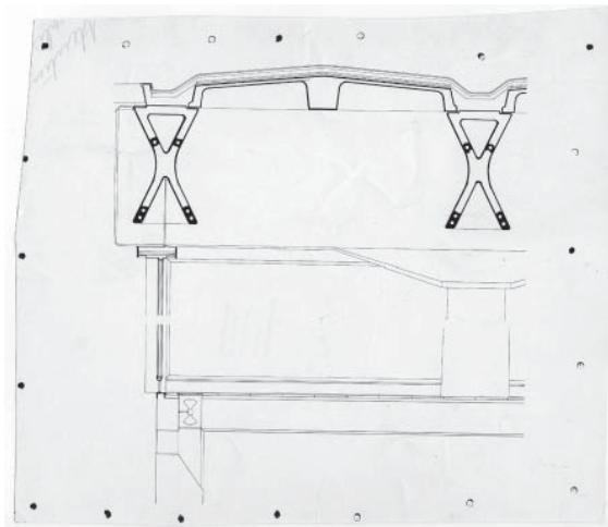
[F2] Iglesia Mater Misericordiae en Baranzate di Bollate (Milán, 1956-58). Detalle de la cubierta con las vigas en X diseñadas por Favini
