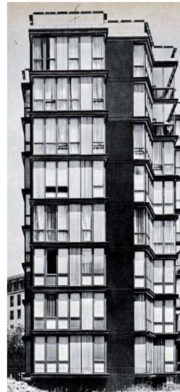
[F12] Bruno Morassutti, Angelo Mangiarotti, Aldo Favini (ingeniero), Edificio de viviendas en via Quadronno (Milán, 1960-62). Los paneles de madera y el vidrio se componen libremente en la fachada en función de las necesidades de las viviendas. Fotografía: Giorgio Casali.
