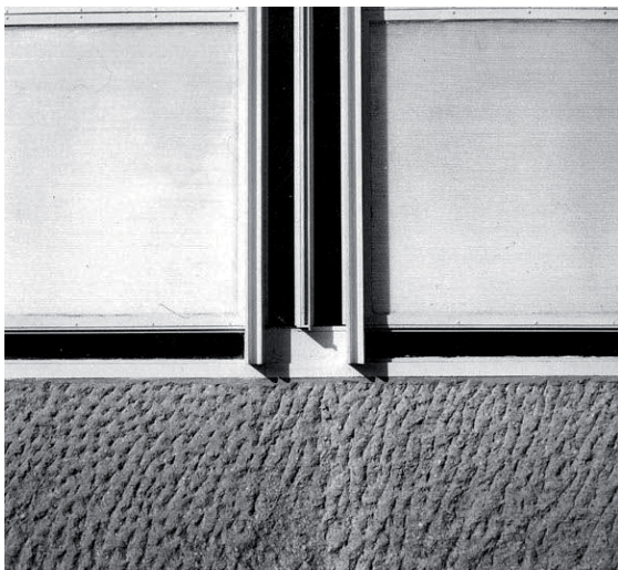
[F3] Bruno Morassutti, Angelo Mangiarotti, Aldo Favini (ingeniero), Iglesia Mater Misericordiae en Baranzate di Bollate (Milán, 1956-58). Detalle del cerramiento en su encuentro con el zócalo. Fotografía: Giorgio Casali
