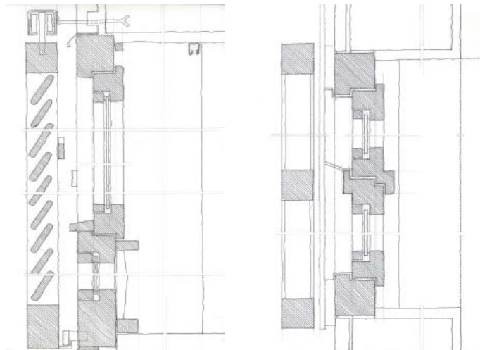
[F10], [F11] Sección y planta de la ventana. © arroyopemjean.
