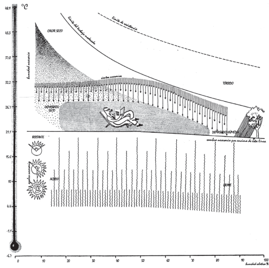
[F11] Victor Olgyay, 'Índice esquemático del bioclima', 1962 [Olgyay, V., Arquitectura y clima, Barcelona, Gustavo Gili, 1998]
