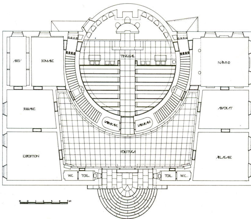
F8 Erik Gunnar Asplund. Tribunal del condado de Lister en Sölversborg. 1917-22. Planta baja
