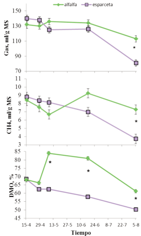
FIGURA 5. Producción de gas y de metano en ml/g MS y desaparición de la materia orgánica (% DMO) in vitro de la alfalfa y de la esparceta según el momento del pastoreo (de abril a agosto). Diferencias entre forrajes en el mismo momento de aprovechamiento, * P < 0,05
