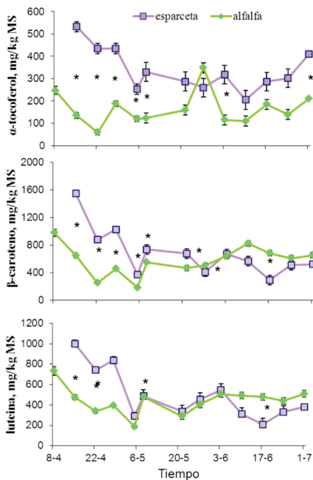
FIGURA 4. Evolución de los contenidos en \alpha -tocoferol, \beta -caroteno y luteína en la alfalfa y esparceta según el momento del pastoreo (de abril a julio). Diferencias entre forrajes en el mismo momento de aprovechamiento, * P < 0,05 .
