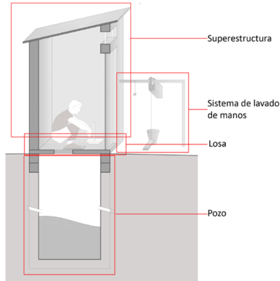
Figura 7. Dibujo de letrina de pozo simple destacando las cuatro partes que la componen Fuente: Adaptado de Esteban-Zazo, A.(Coord.), Mancebo-Piqueras, J.A. & Zapico, A., (2014). Affordable Sanitation Products, Choo Bora na Mazingira Safi. Kongwa Distric (p 11).
