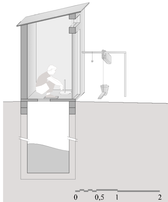
Figura 3. Letrina de pozo simple
