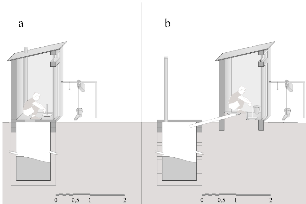
Figura 4. (a) Letrina ventilada mejorada con pozo dentro (b) Letrina tradicional ventilada mejorada con arrastre de agua y pozo fuera
