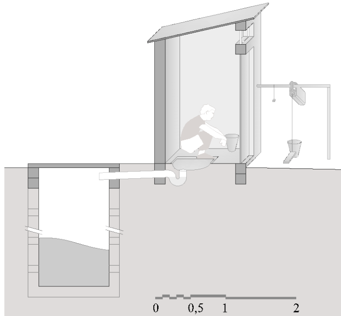
Figura 5. Letrina con sifón
