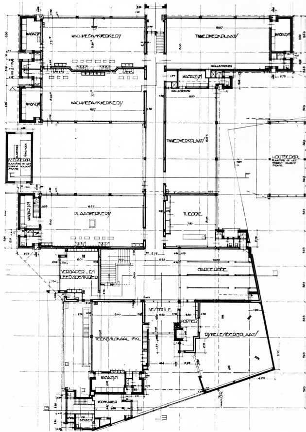
Derde Ambachtsschool, Scheveningen, primer proyecto. Perspectiva, planta.
