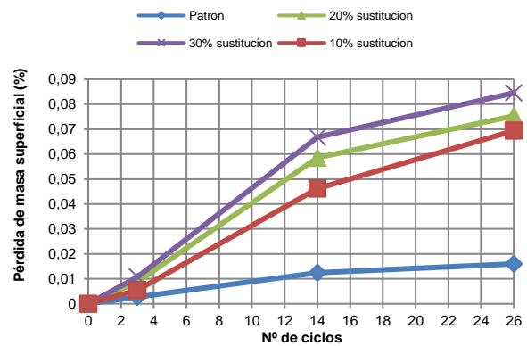
Fig. 5: Pérdida de masa media por ciclos.
