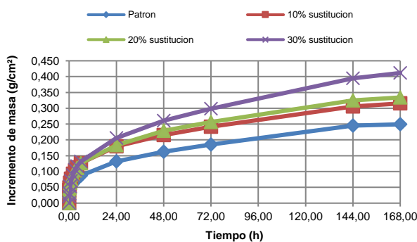
Fig. 4. Incremento de masa medio por absorción capilar (g/cm 2 ).
