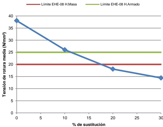
Fig. 1. Comparación de la tensión de rotura media a compresión a 28 días con los límites de la EHE 08.
