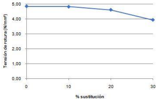
Fig. 2. Tensión de rotura de probetas a flexión a 28 días.
