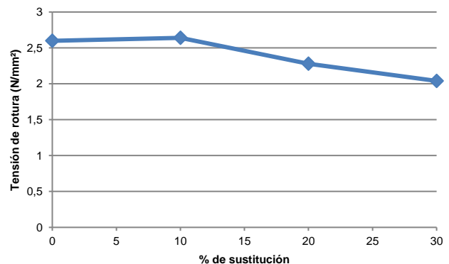
Fig. 3. Tensión de rotura de probetas a tracción a 28 días.
