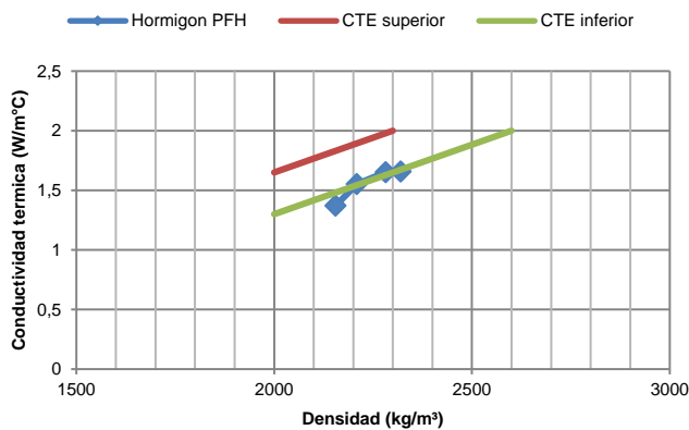
Fig. 7: Comparación de conductividad térmica de los hormigones con el catálogo técnico de elementos constructivos del CTE.
