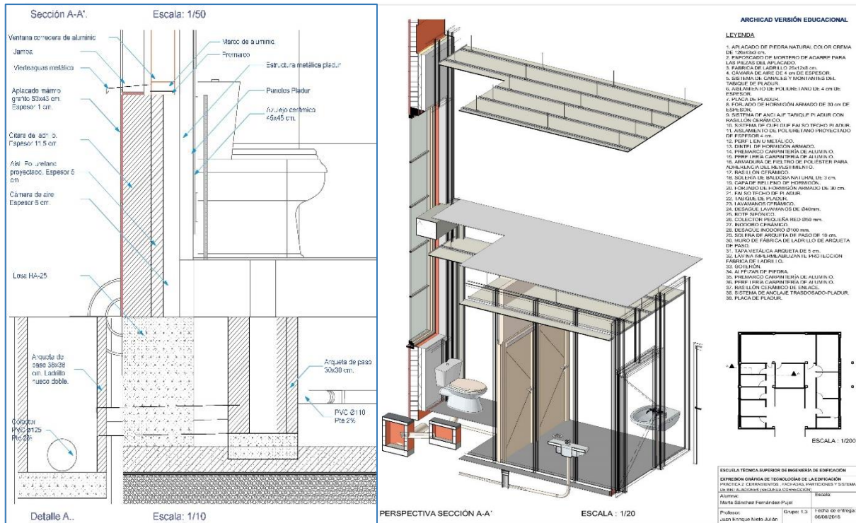
Fig. 5. Análisis de sistemas de divisiones, falsos techos e Instalaciones en la zona de aseos. Detalles Axonométricos realizados con ArchiCAD 19. Alumno autor: Marta Sánchez
