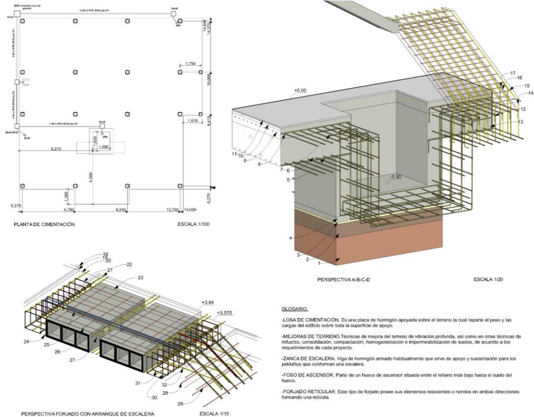
Fig. 4. Arranque y desembarco de la zanca de escalera, con disposición de las armaduras. Detalles Axonométricos realizados con ArchiCAD 19. Alumno autor: Marta Sánchez.
