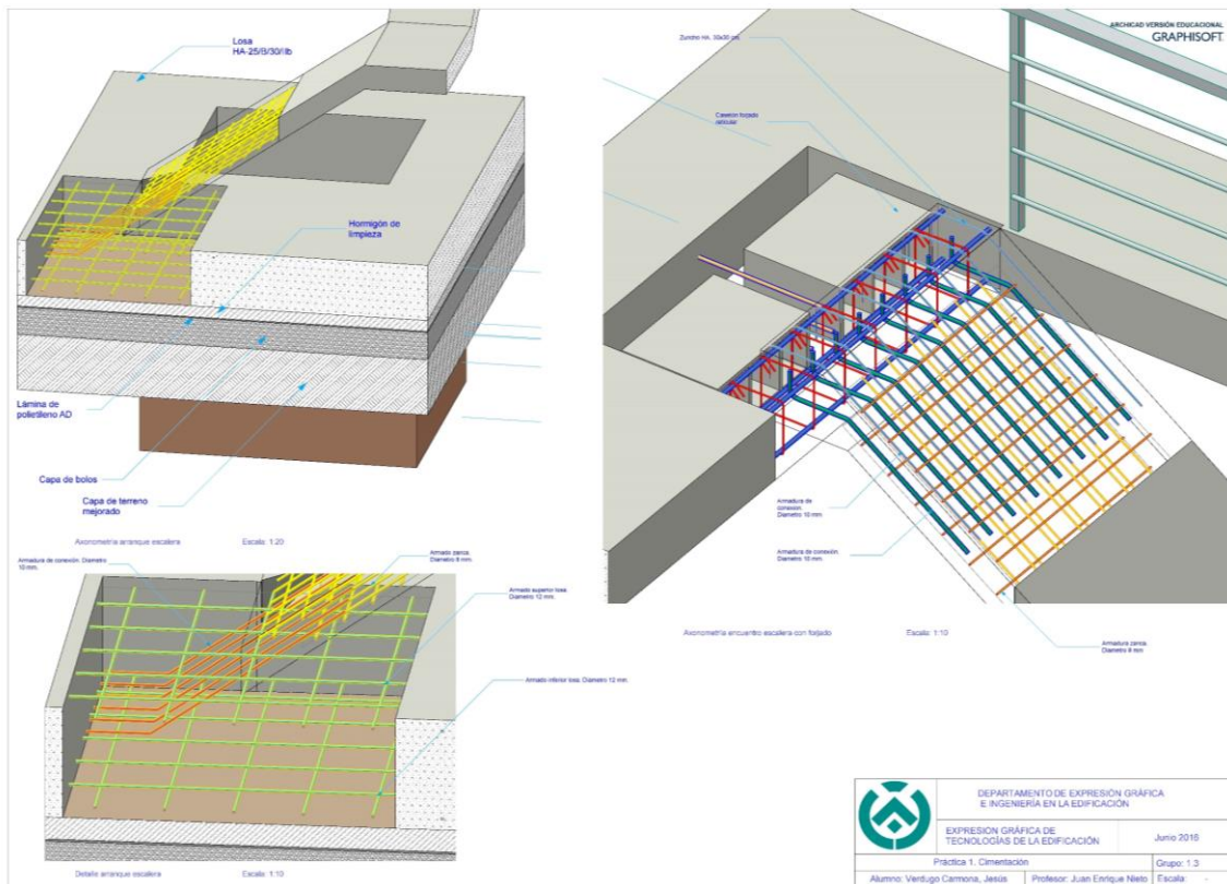
Fig. 3. Arranque y desembarco de la escalera, con el análisis del reparto de las armaduras. Detalles Axonométricos realizados con ArchiCAD 19. Alumno autor: Jesús Verduo.
