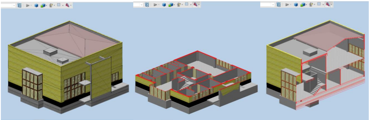
Fig. 2. Modelado del edificio, empleando el software BIM Allplan. Explorado en archivo 3D.pdf.
