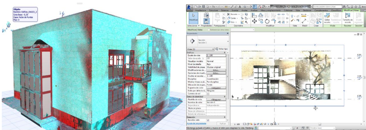
Fig. 7.a. Inserción en ArchiCAD de la Nube de puntos procedente del escaneado del edificio. b. Base referencial para un modelado fiel del edificio (Vista Alzado de la N. Puntos en Revit).
