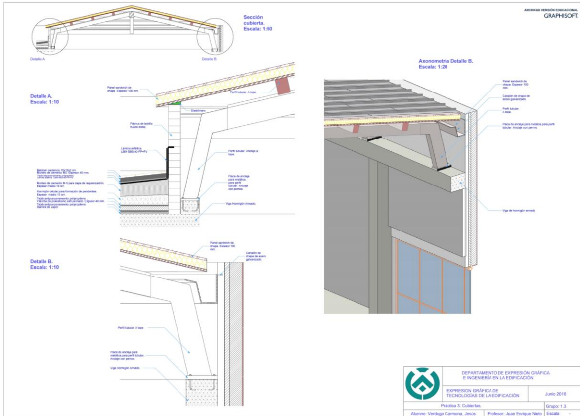
Fig. 8. Práctica III de EGTE. Análisis de sistemas de Cubrición. Detalles realizados con ArchiCAD 19. Alumno: Jesús Verdugo.
