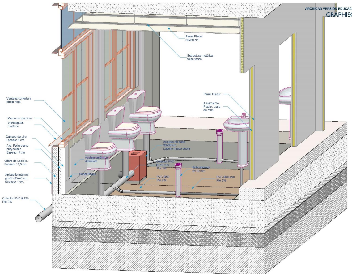
Fig. 6. Análisis de sistemas de divisiones, falsos techos e Instalaciones en la zona de aseos. Detalles Axonométricos realizados con ArchiCAD 19. Alumno autor: Jesús Verdugo.
