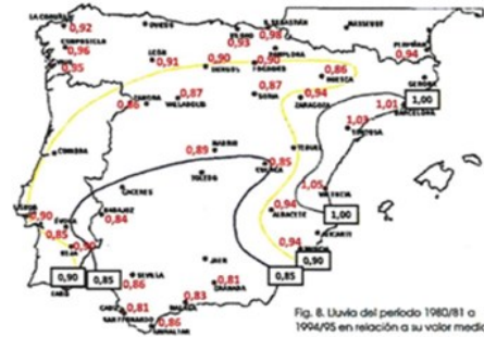
Figura 24: Pluviometría por periodos en relación con su valor medio. Fuente: J.R. Témez, 2005
